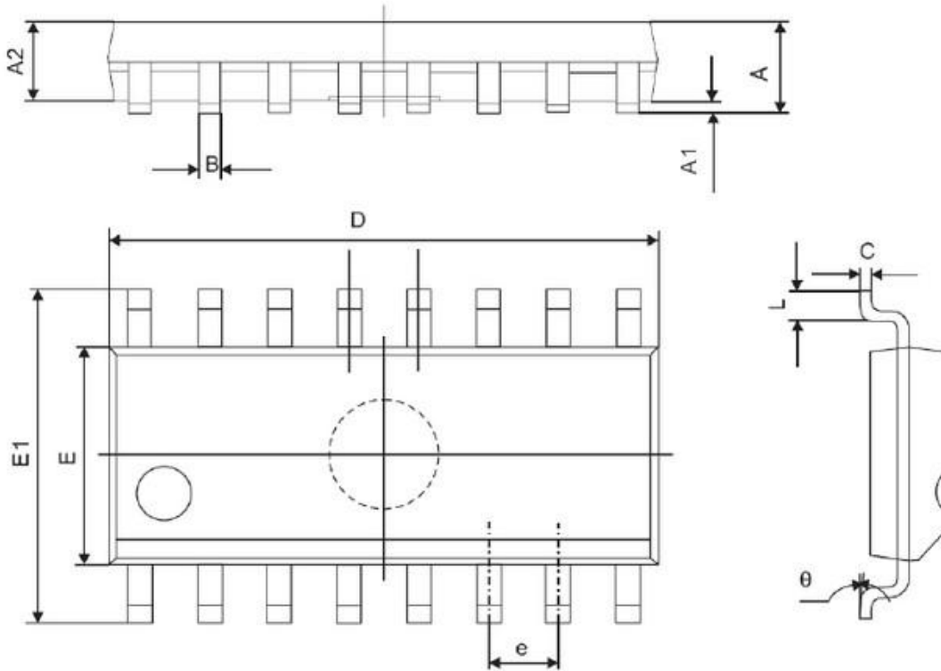
SOP-16
