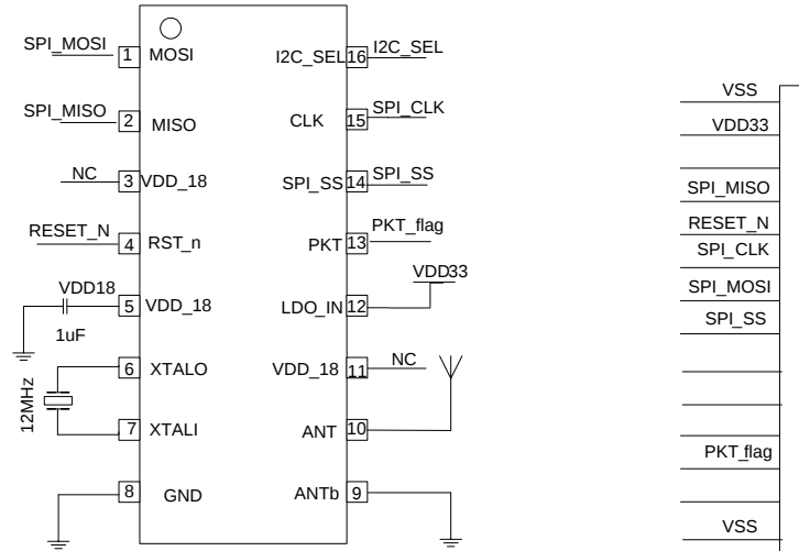
Figure 1. LT8901 典型应用电路
