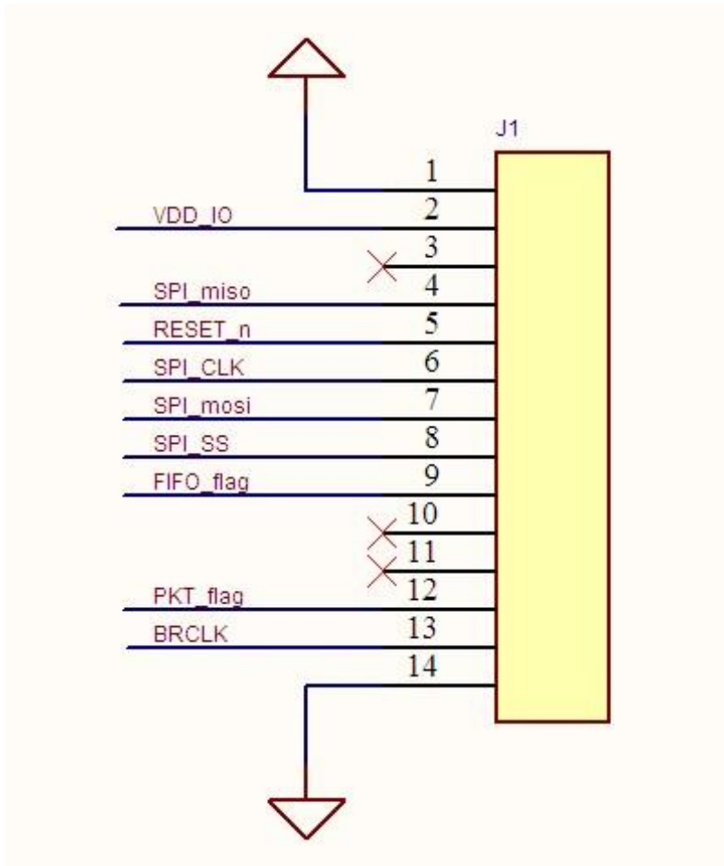
EVB PIN 定义
